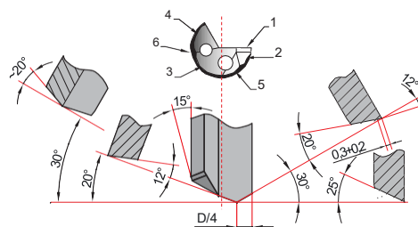
Esquema de afiação standard de brocas monolabiais com \varnothing = 5 a 30mm
