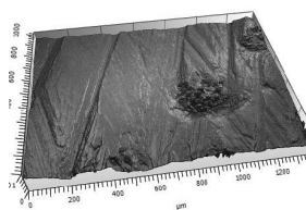
Estrutura após 10 peças
